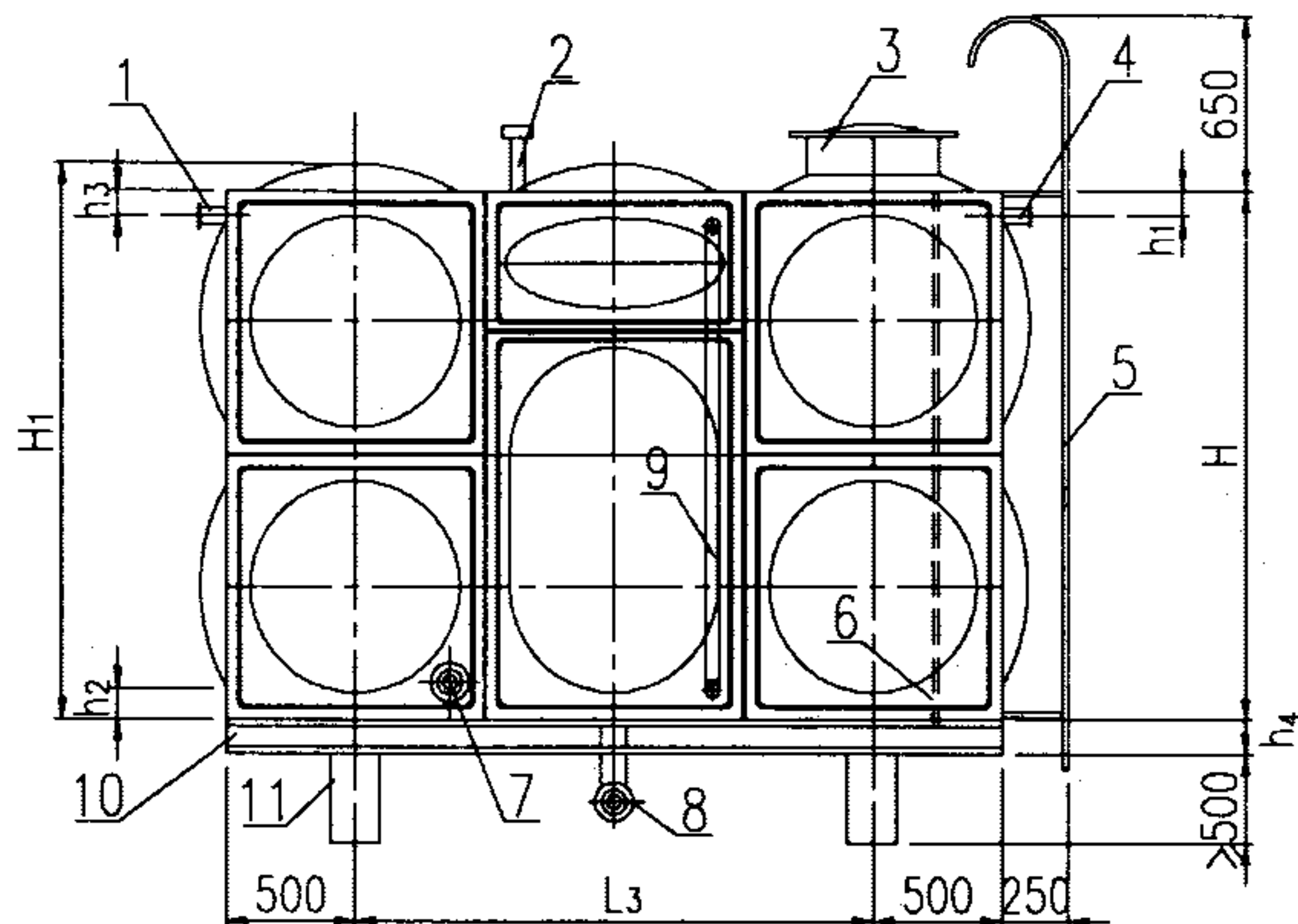
立面图
