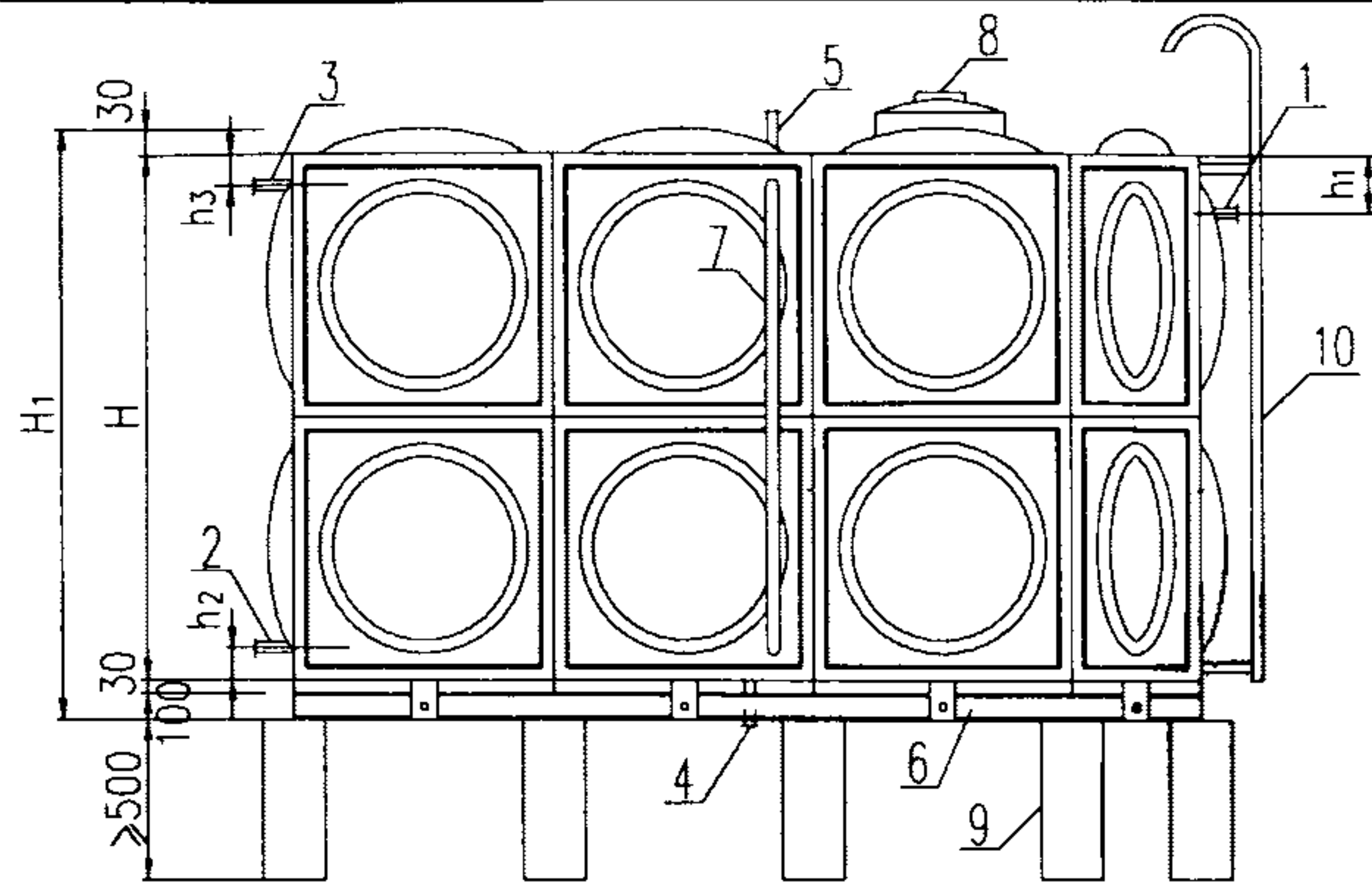
立面图
