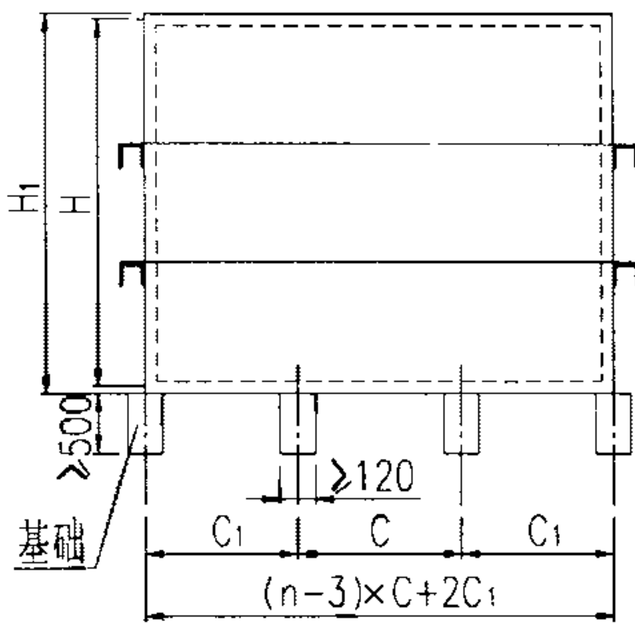
立面图
