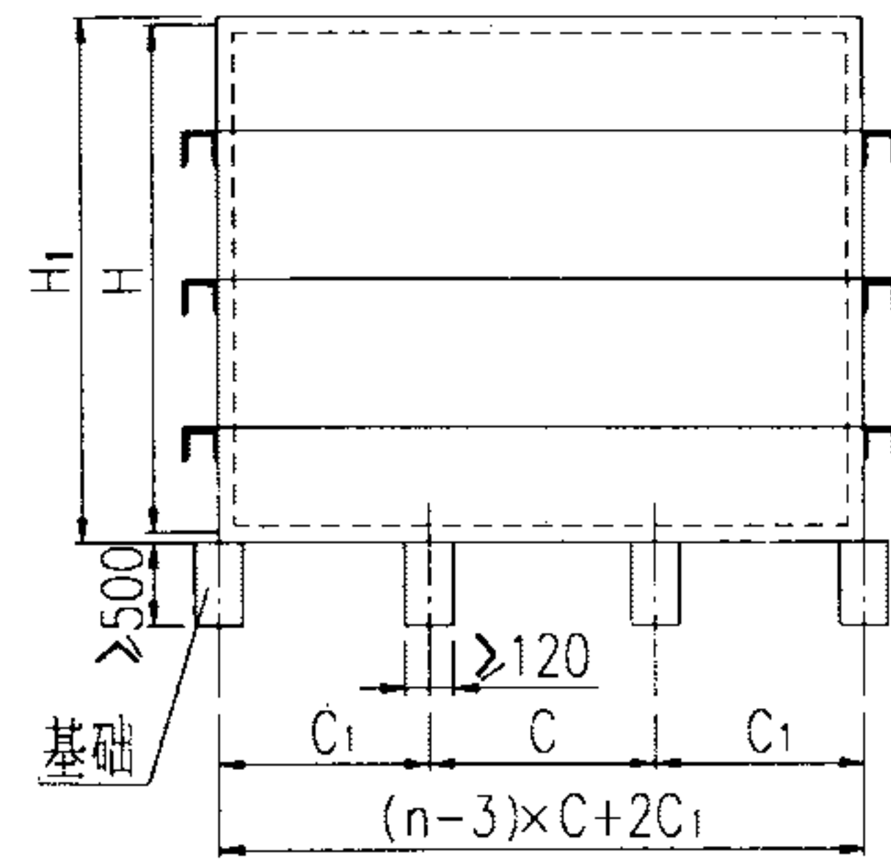
立面图
