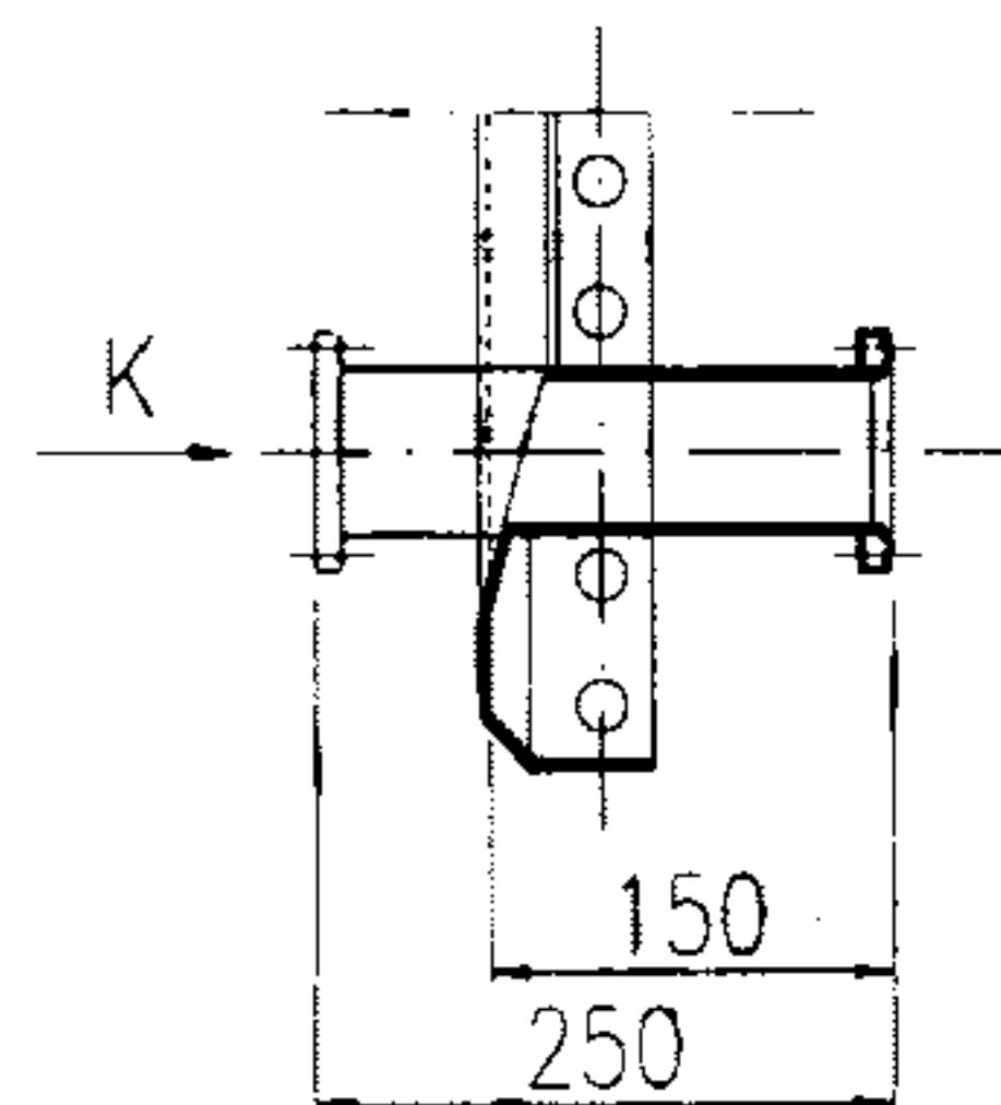
开孔接管图
