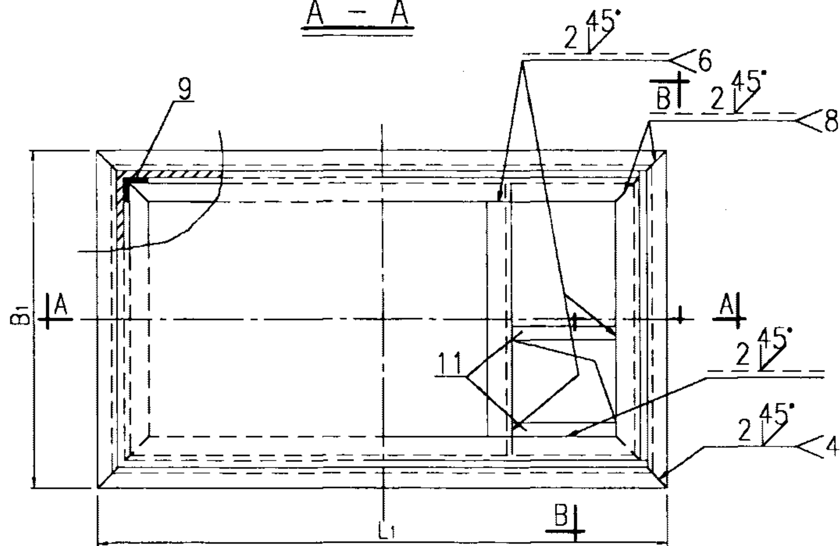
平面图
