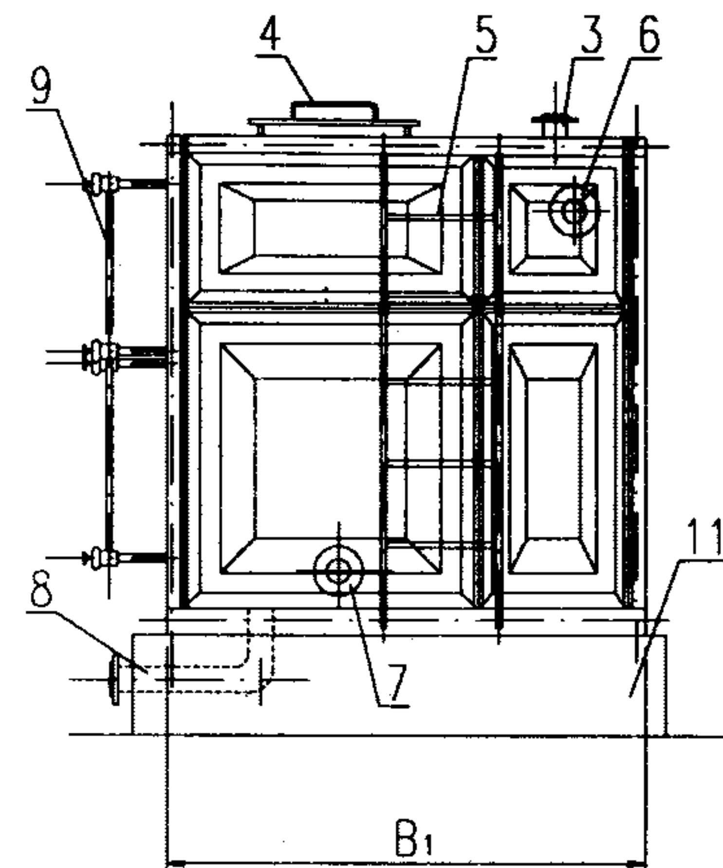
侧立面图
