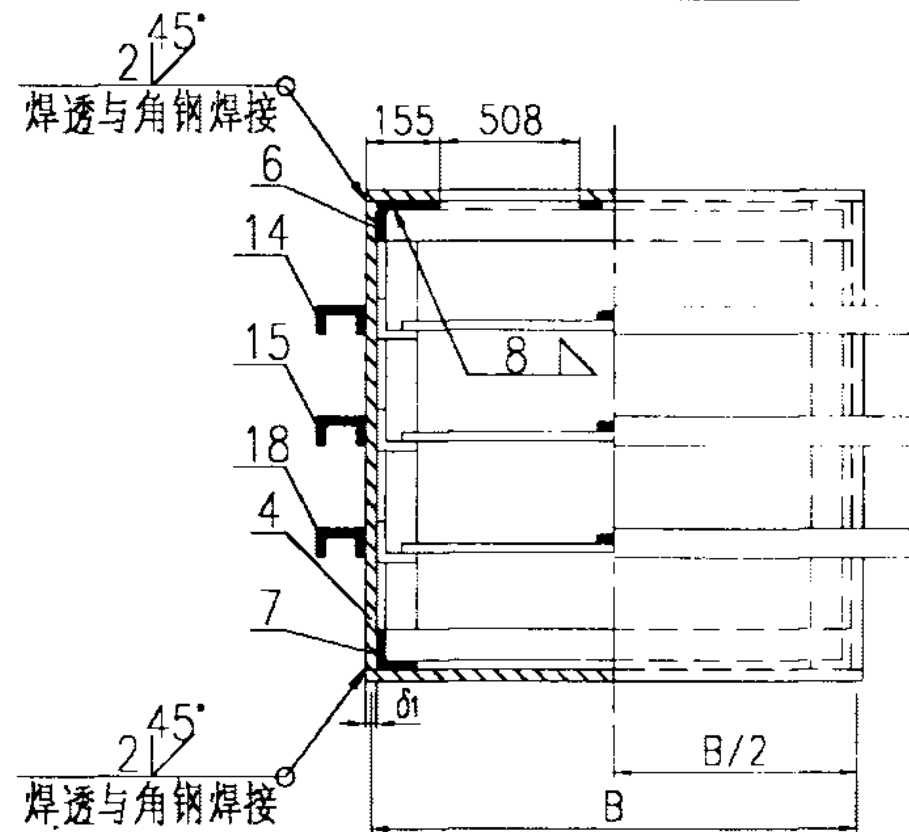
B - B
