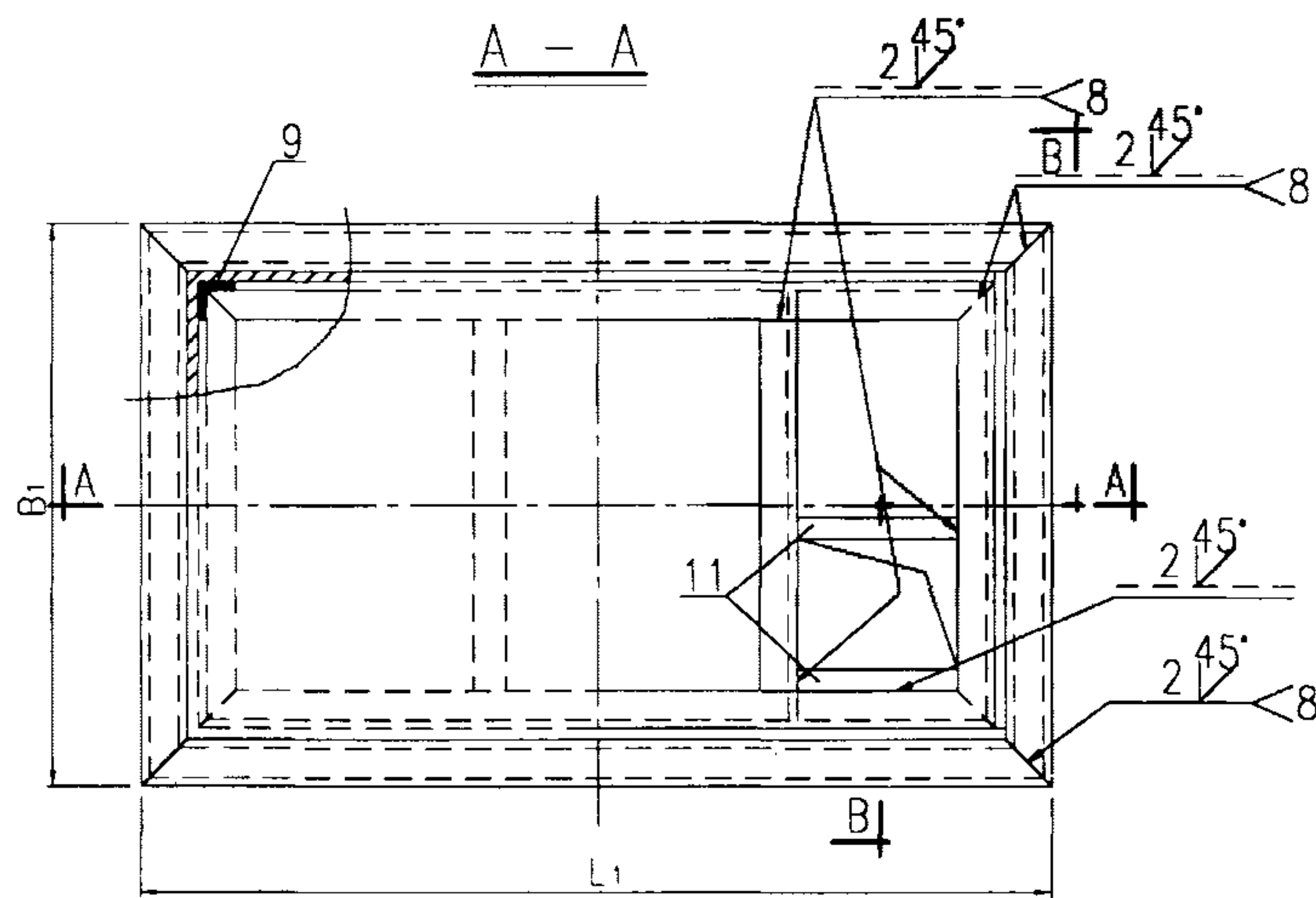
平面图
