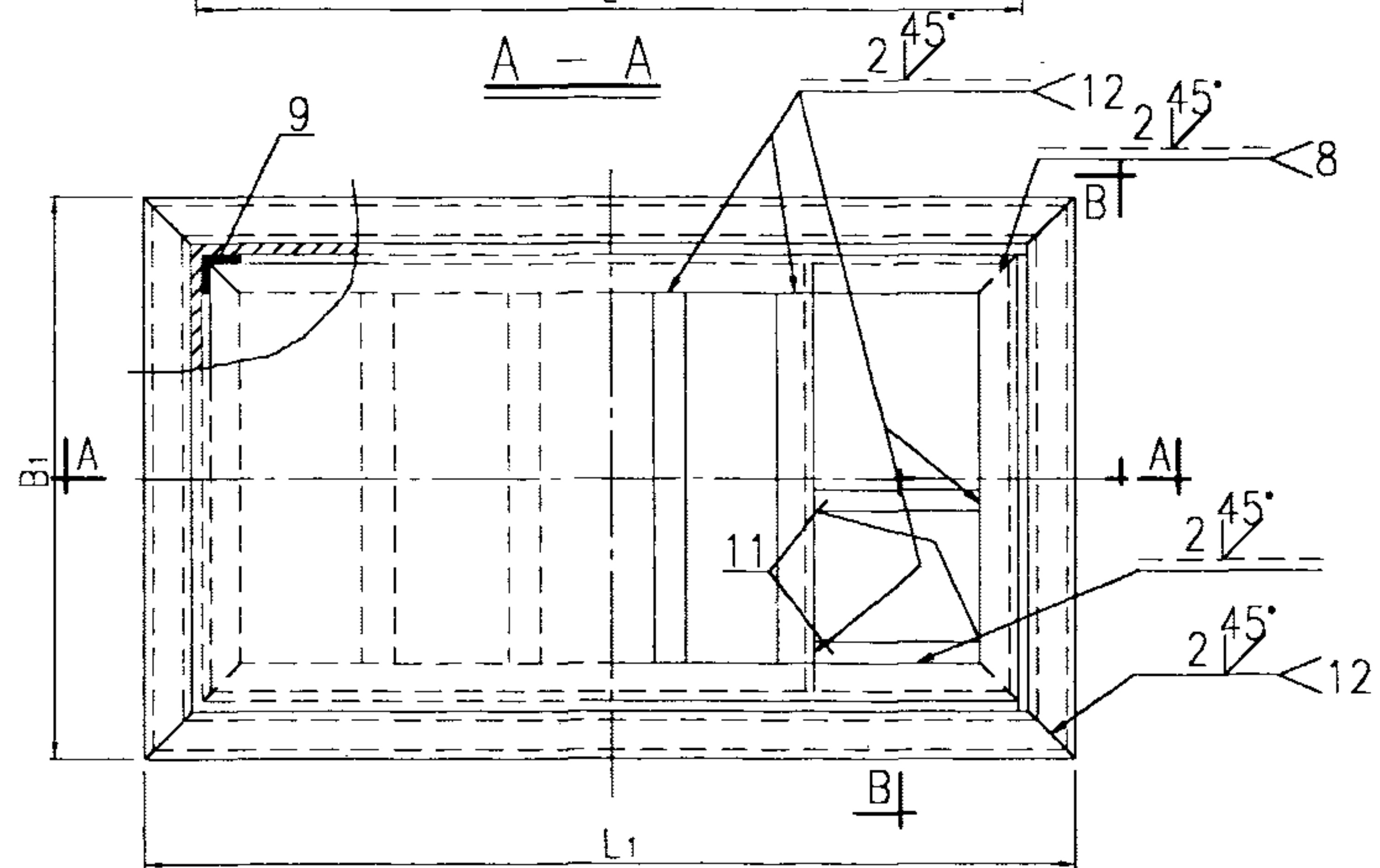
平面图
