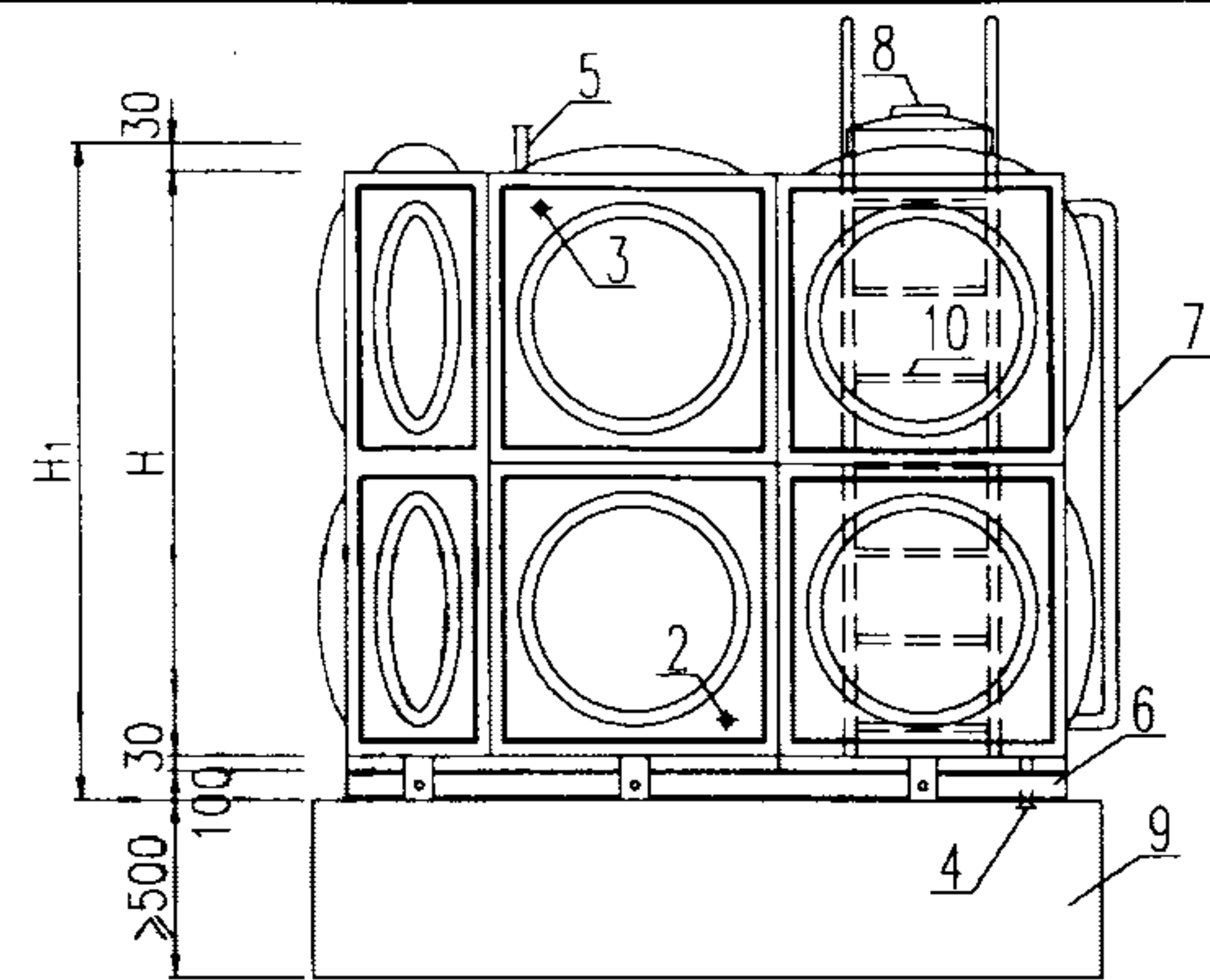
侧立面图
