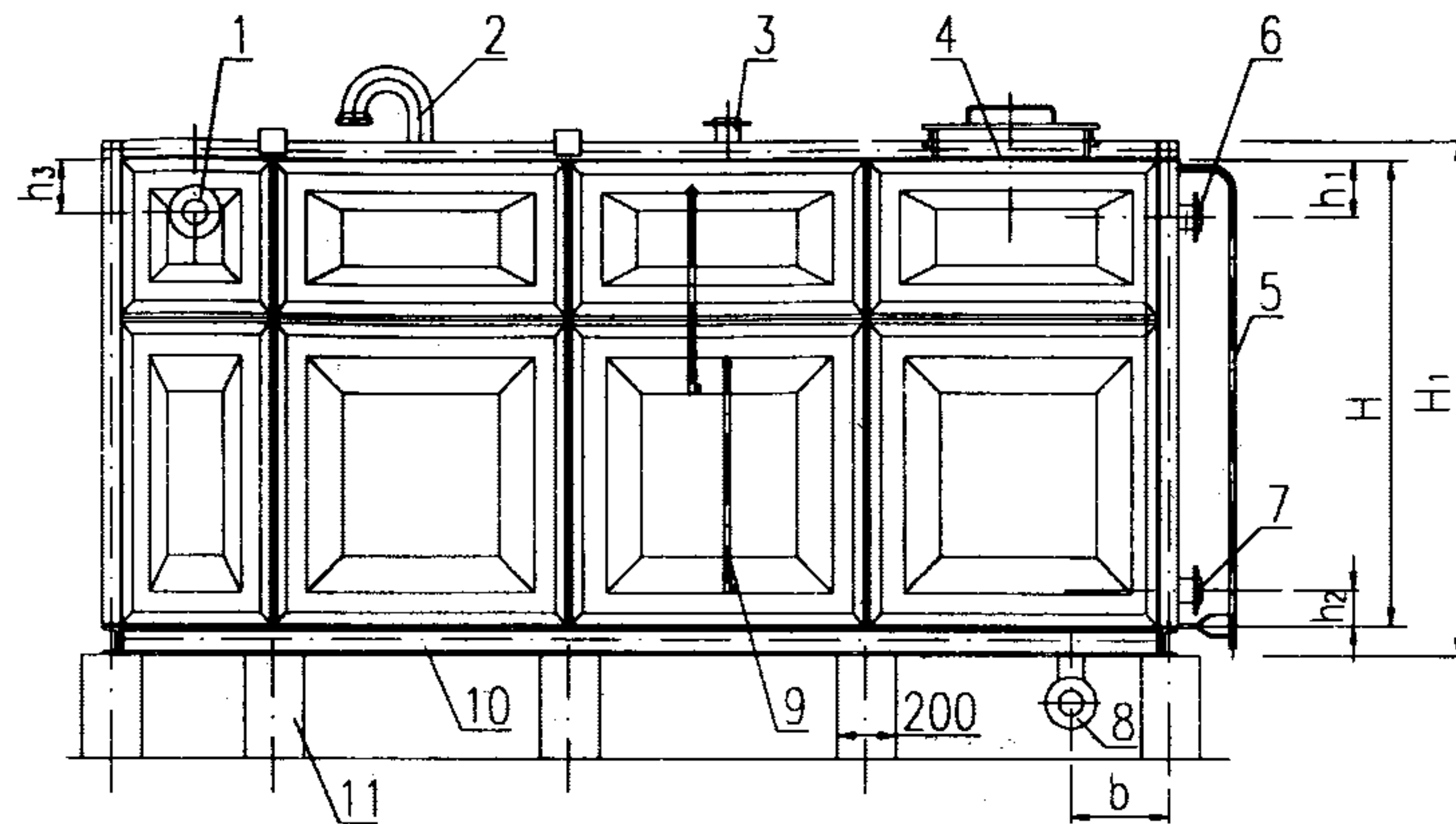
立面图
