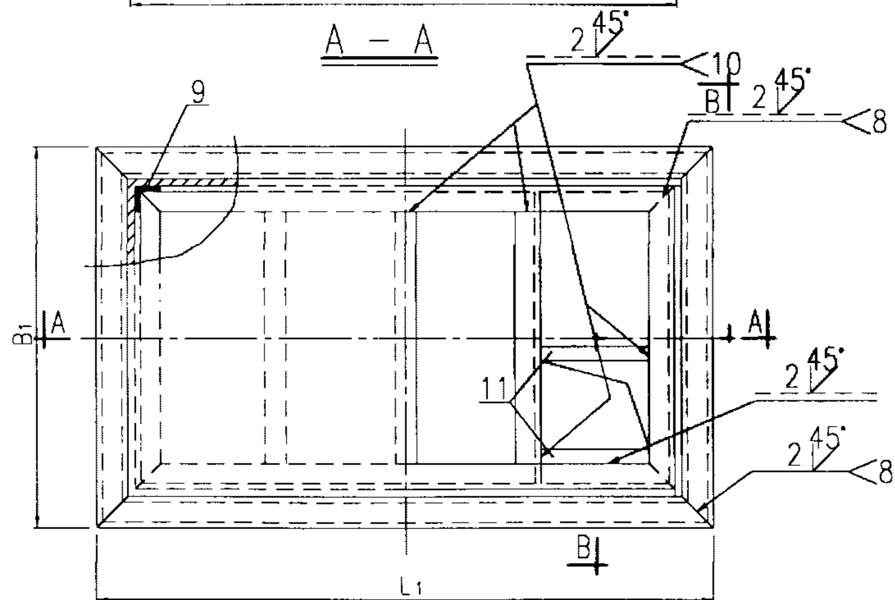
平面图
