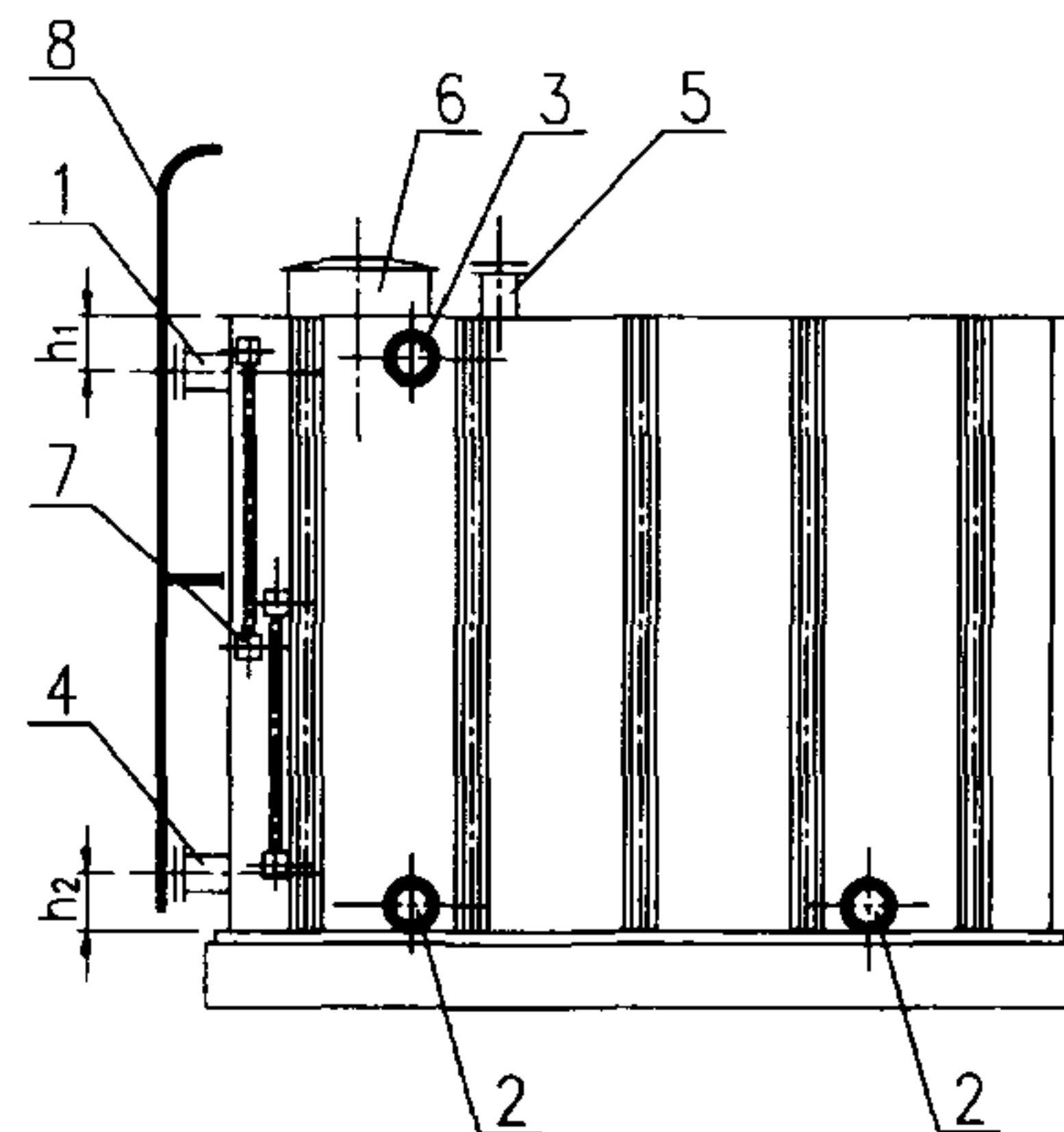
侧立面图
