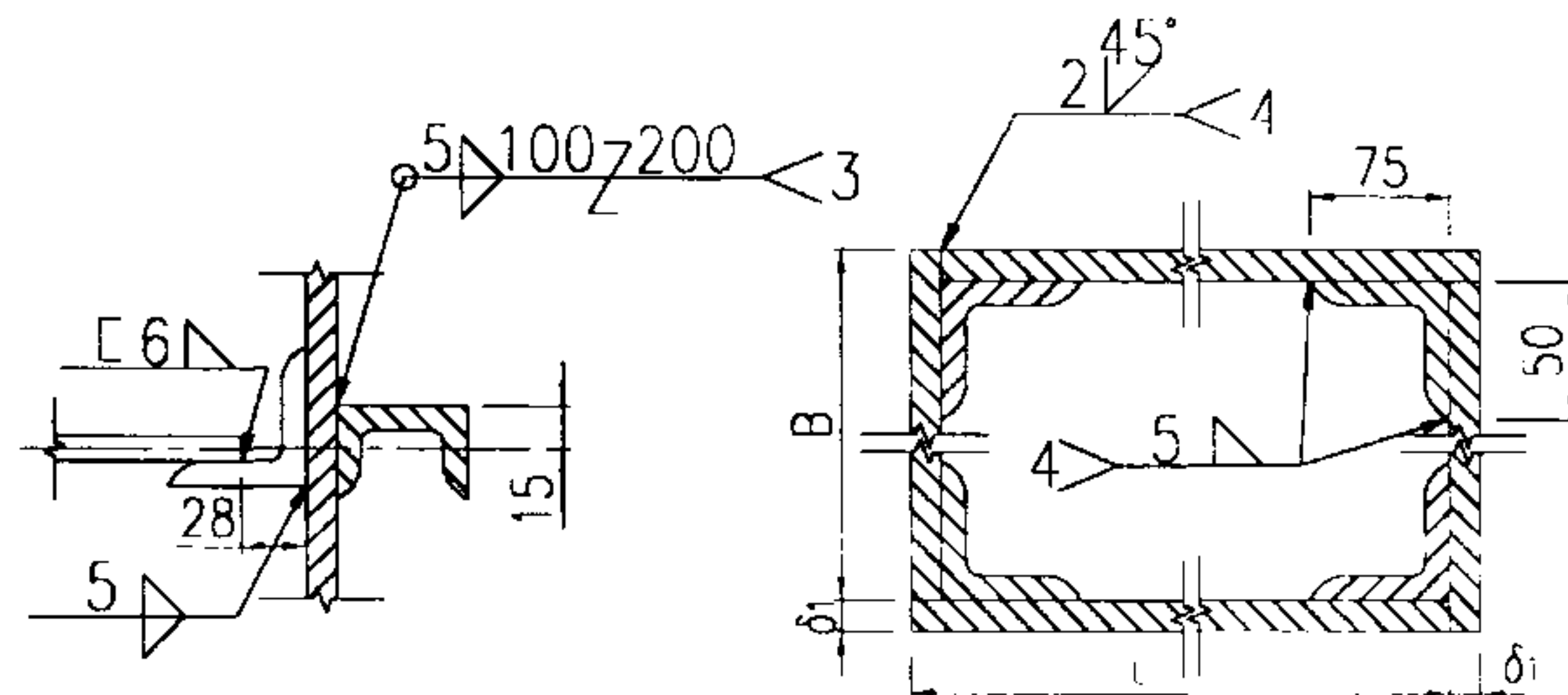
箱壁拼板图
