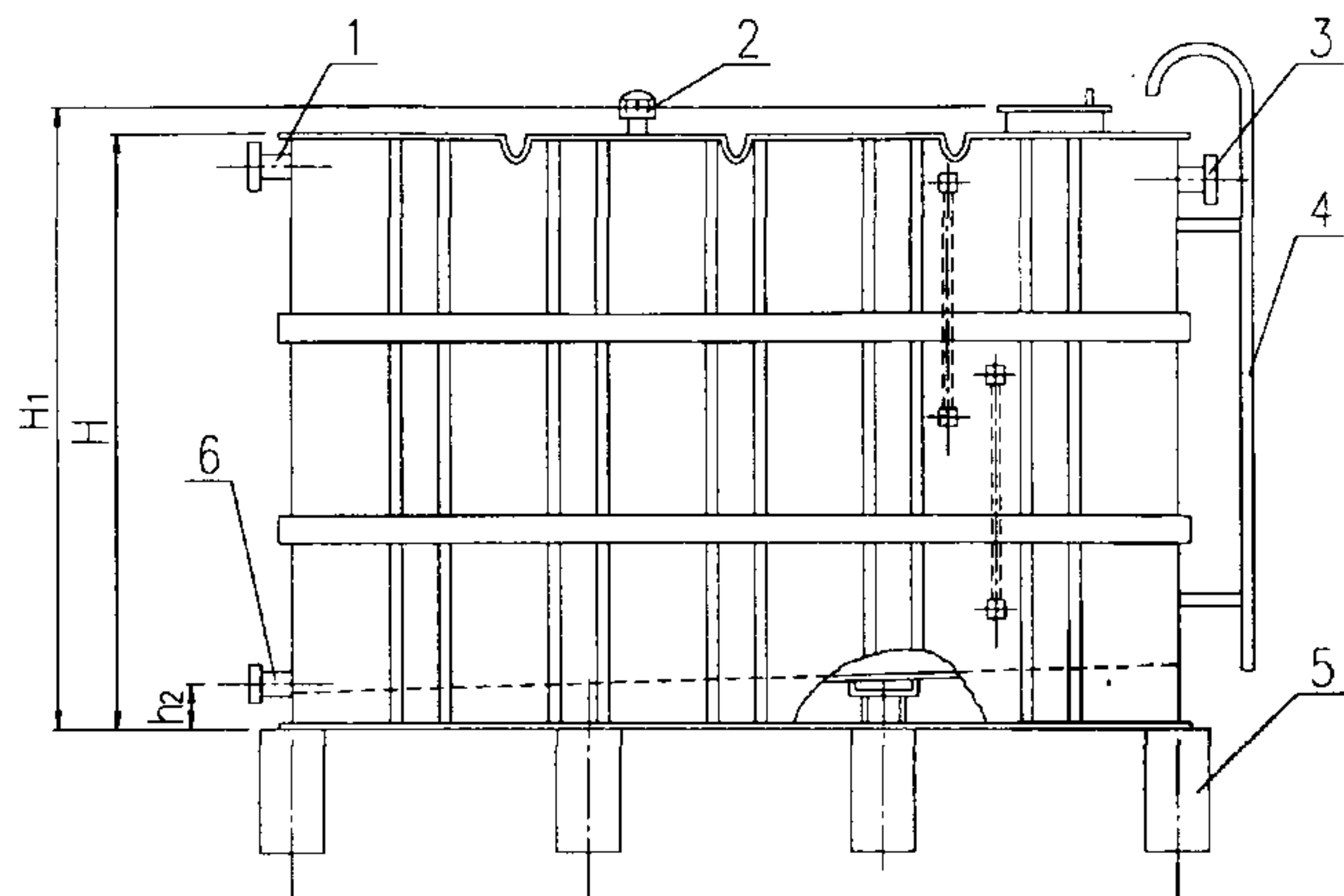
立面图
