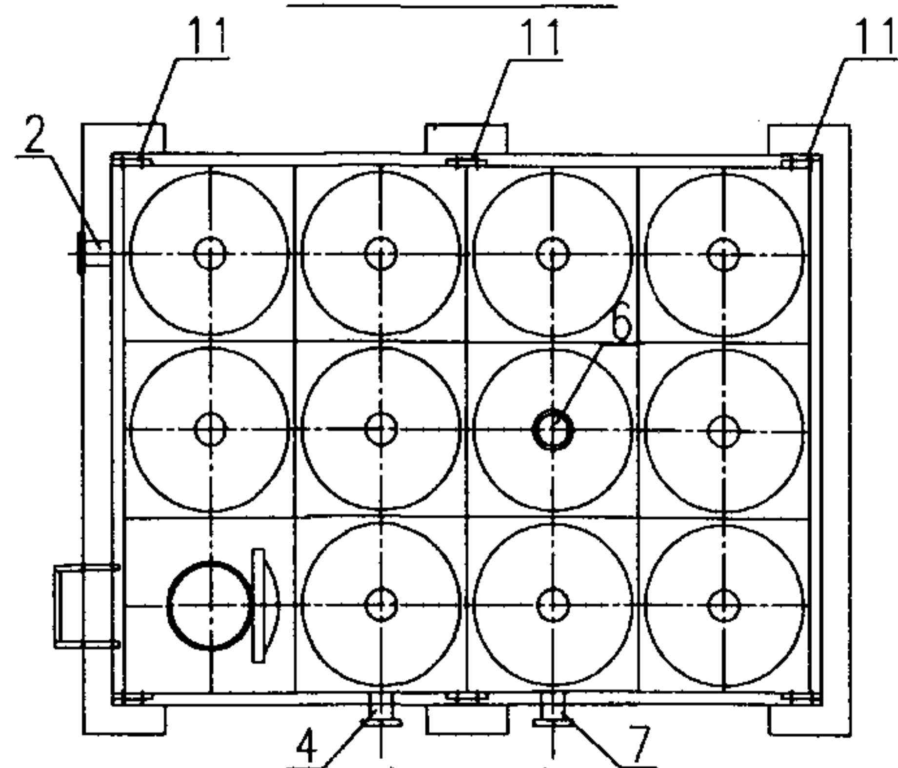
平面图
