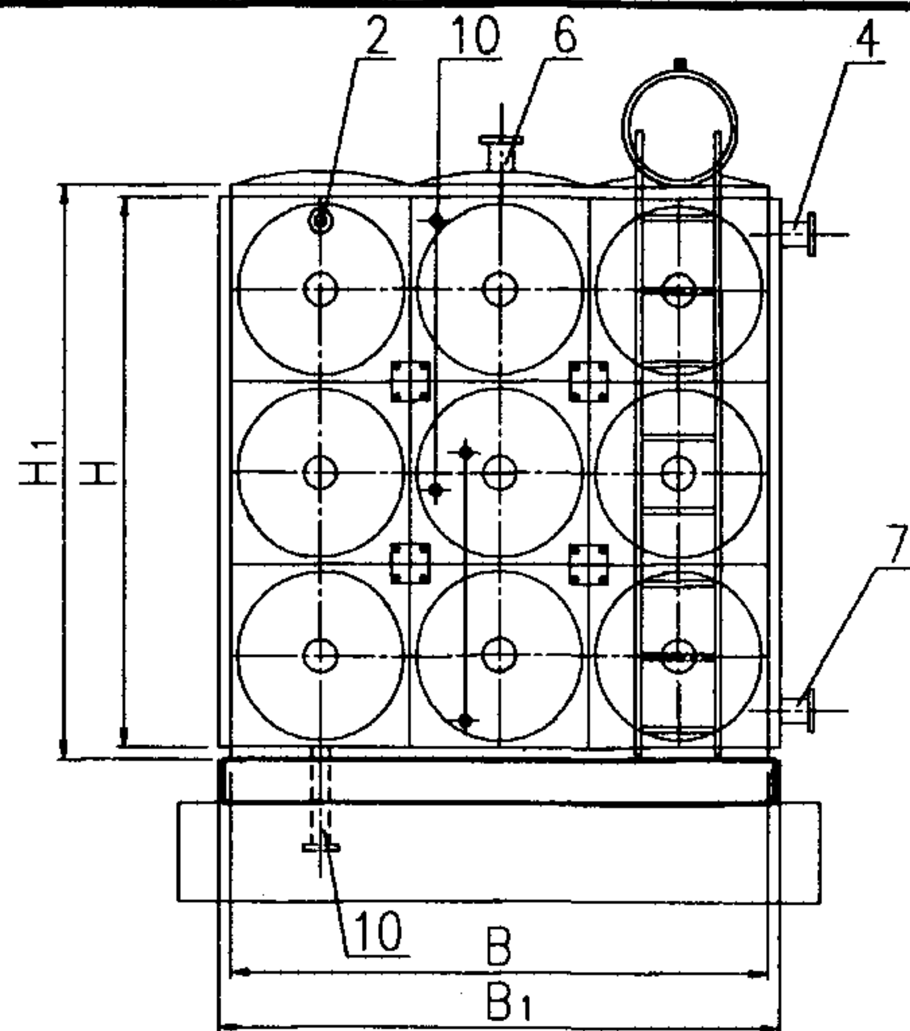
侧立面图
