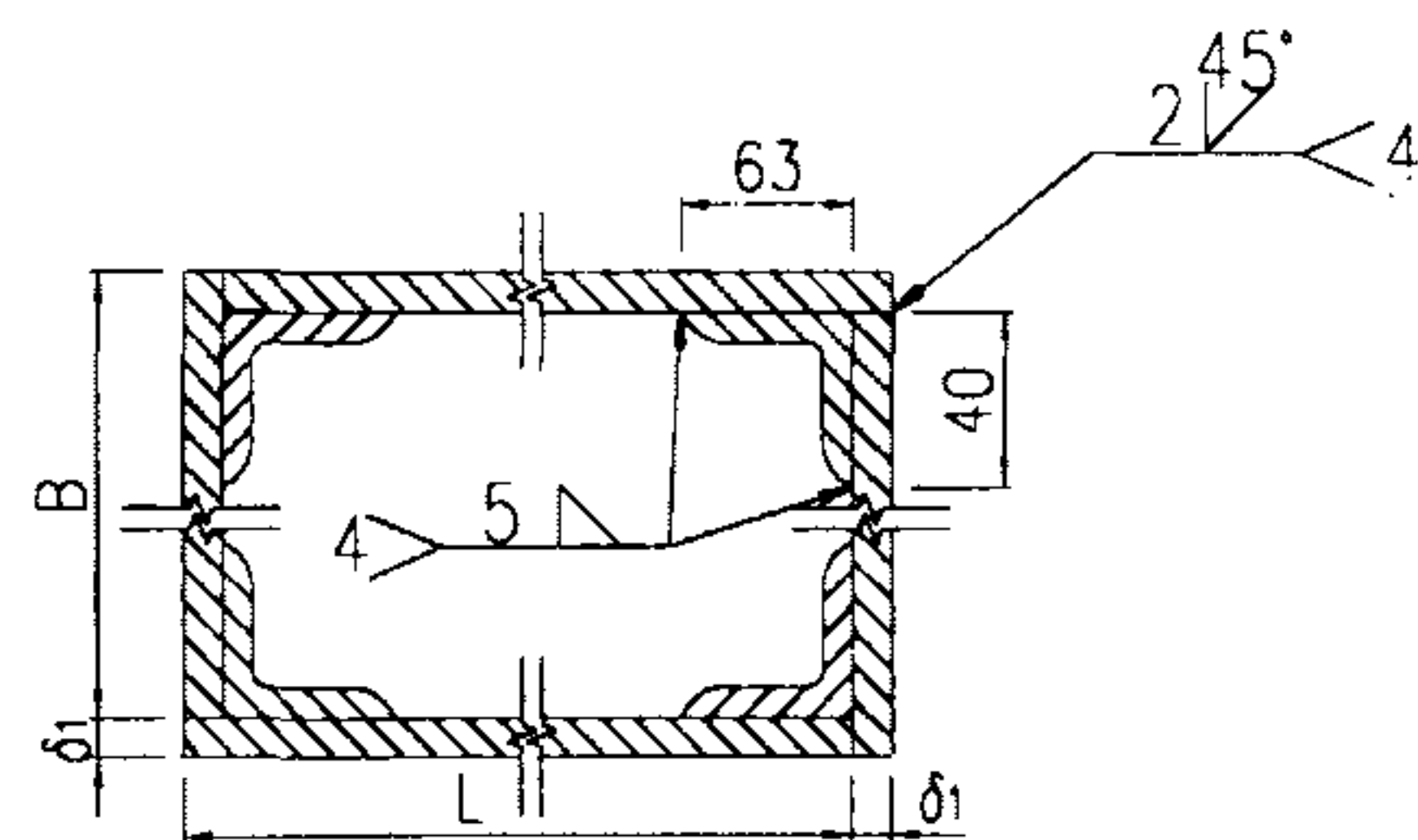
箱壁拼板图
