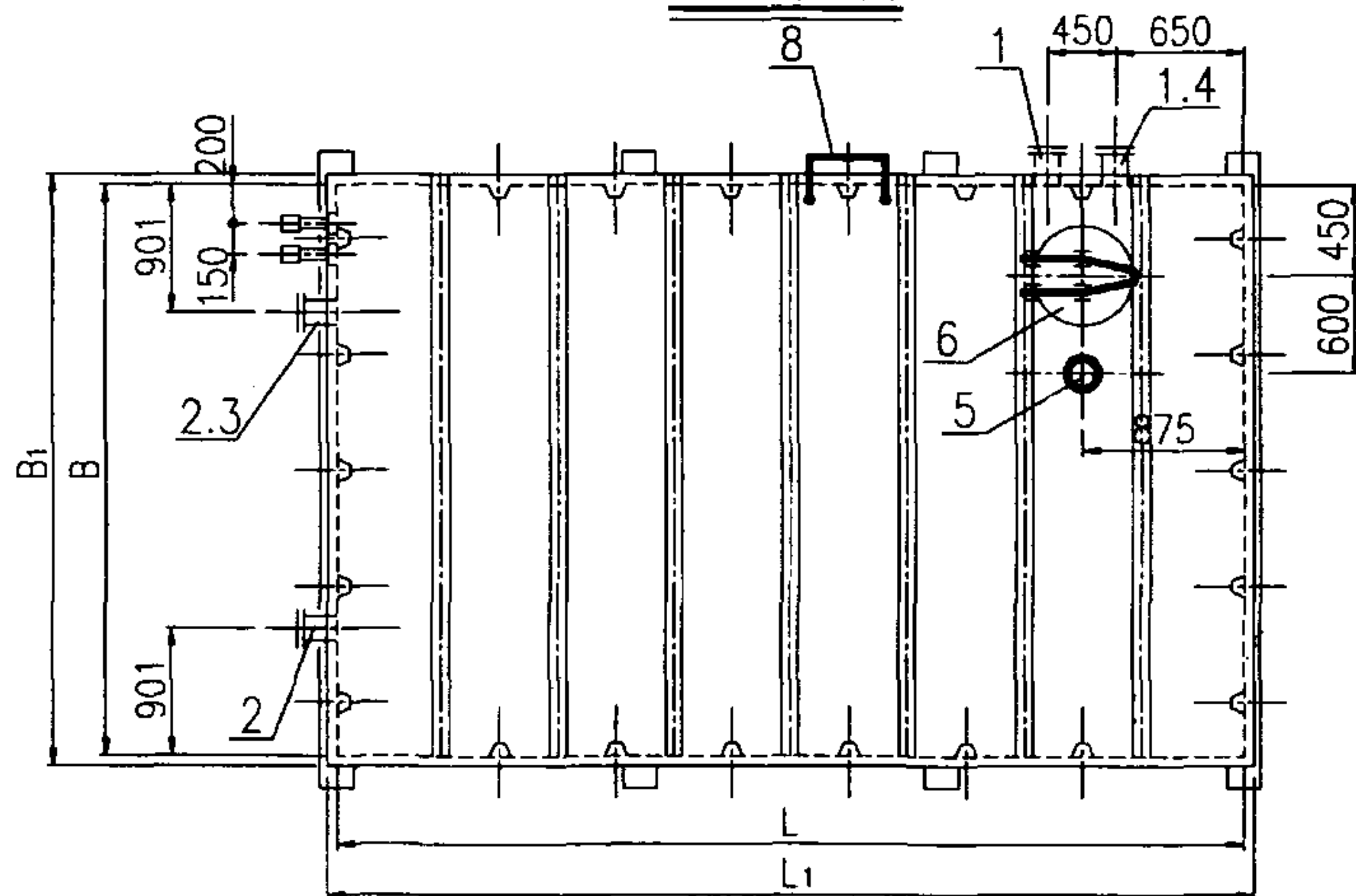
平面图
