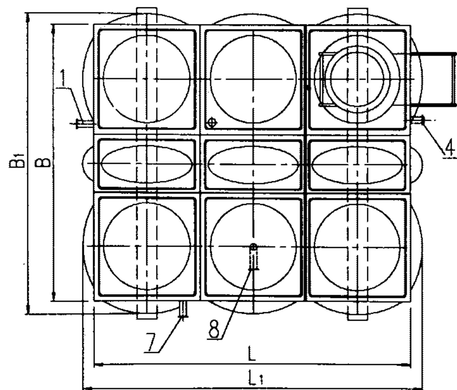
平面图
