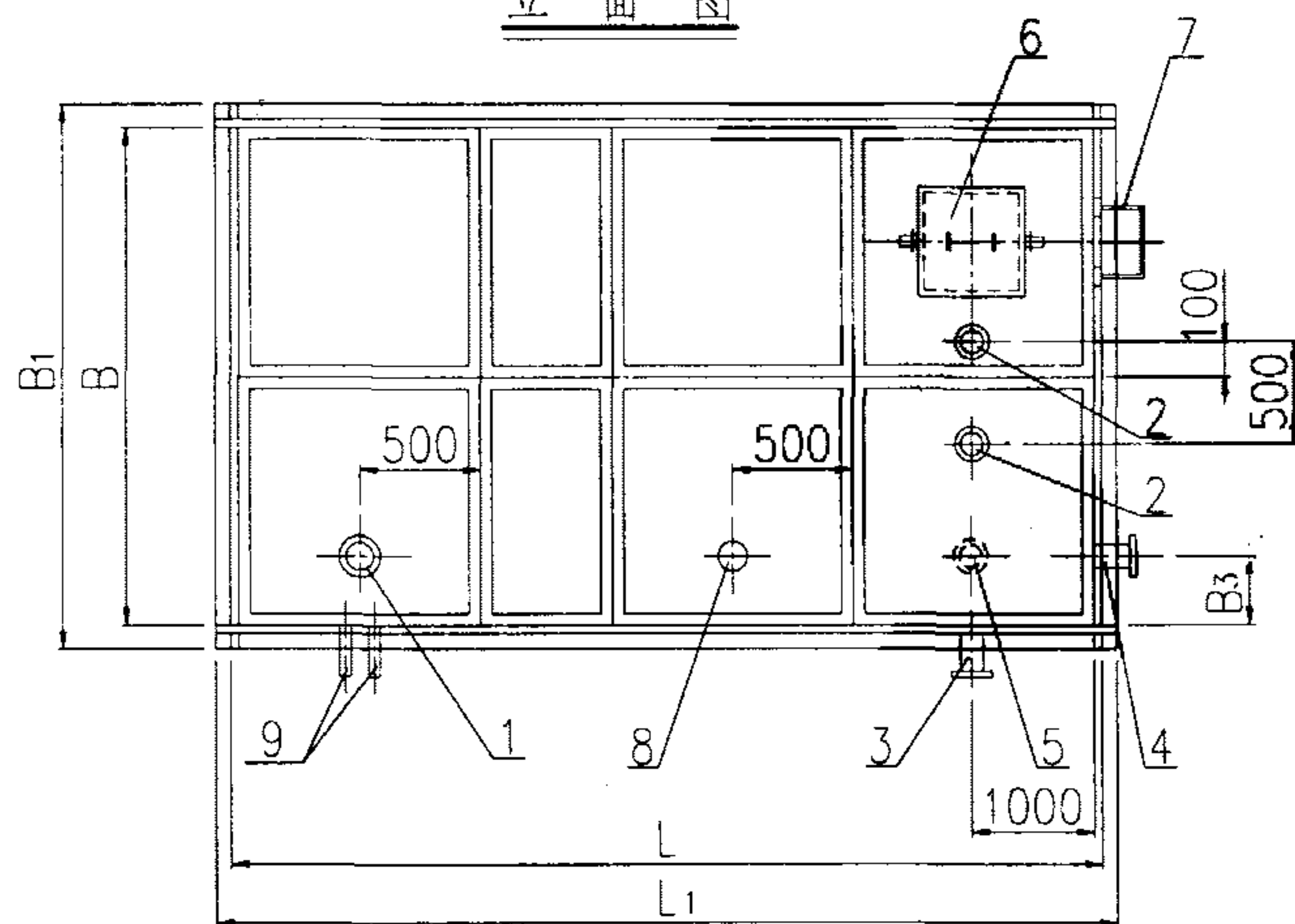
平面图
