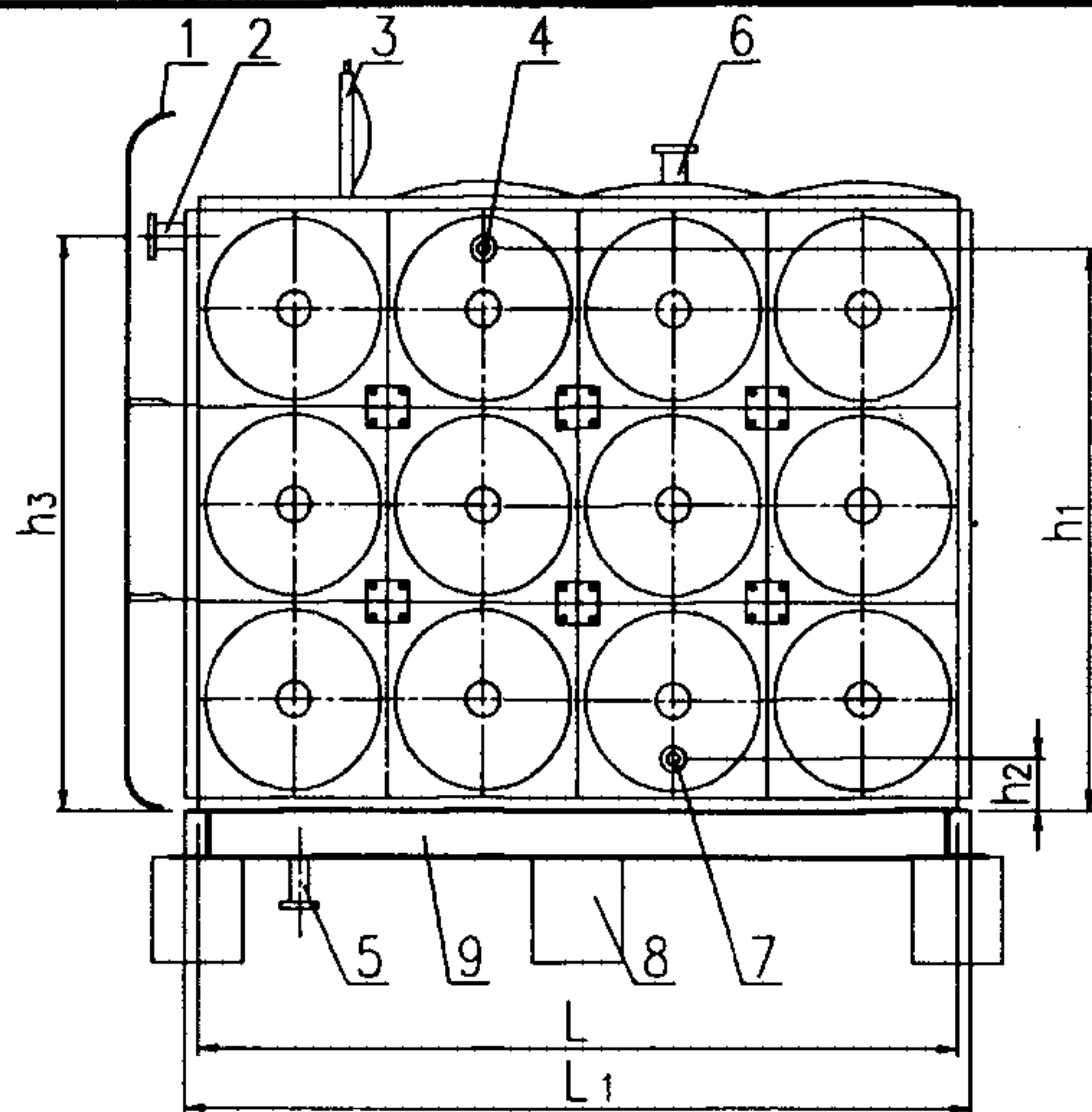
正立面图
